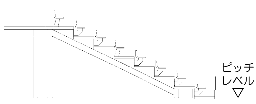
観客席断図
